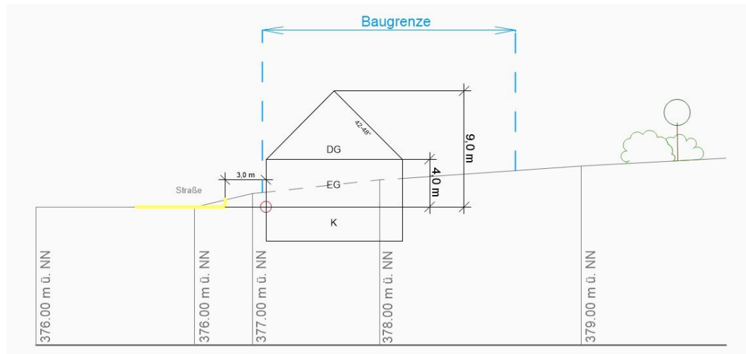
Prinzipschnitt West-Ost
